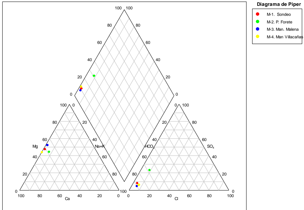
Figura 6. Diagrama de Piper-Hill-Langelier de las 4 muestras
