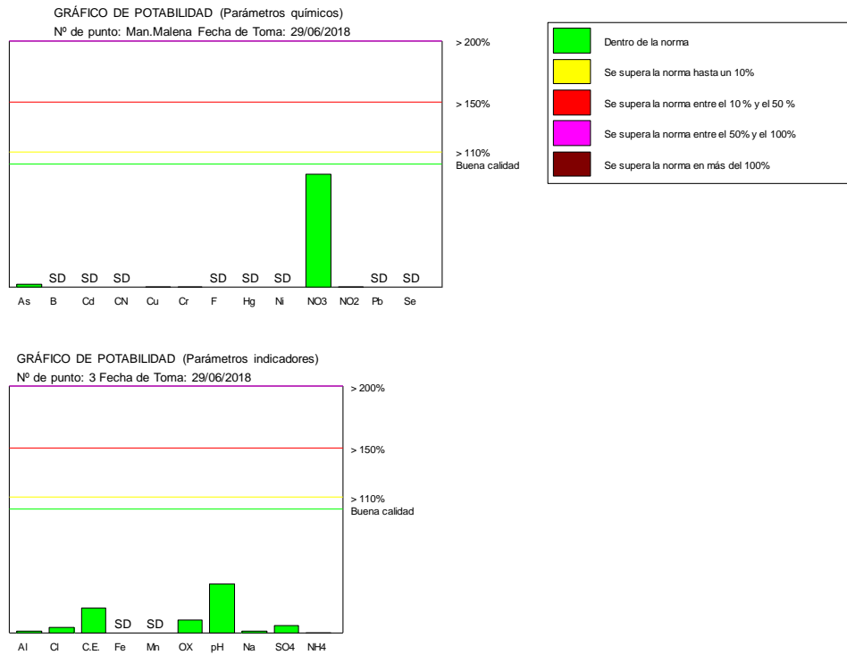
Figura 15. Gráfico de potabilidad del manantial Malena del Encaño
