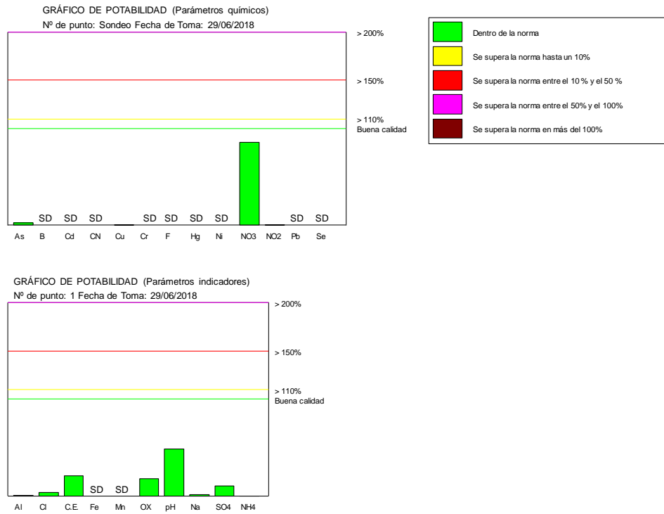
Figura 13. Gráfico de potabilidad del Sondeo
