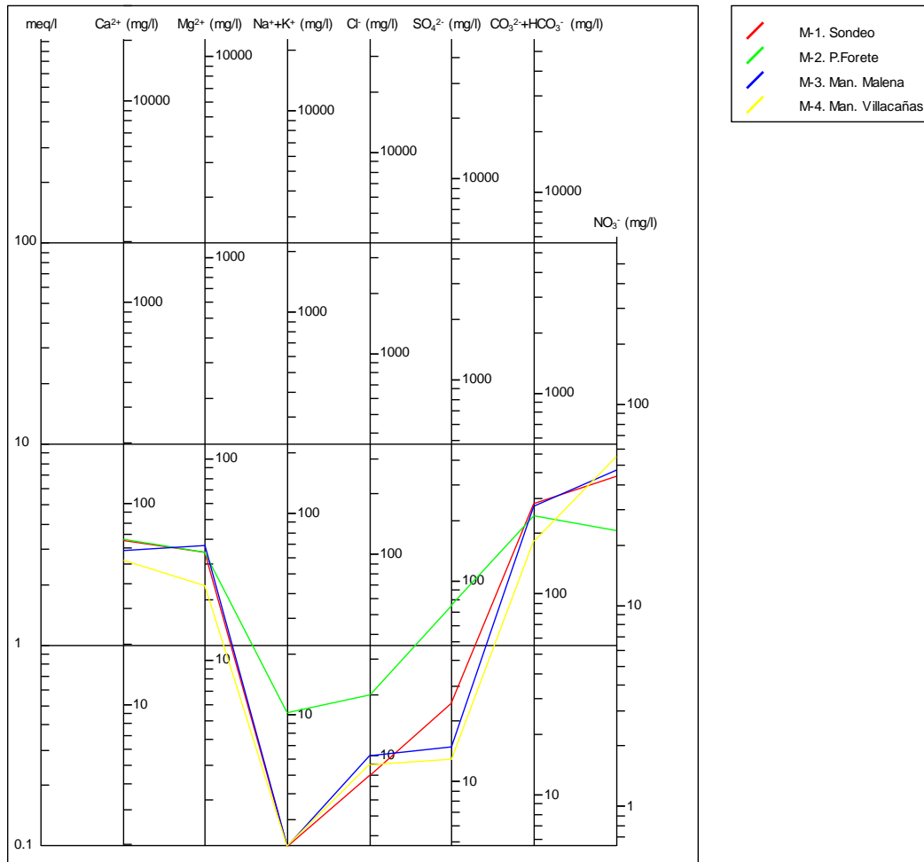
Figura 8. Diagrama de Schöeller de las 4 muestras
