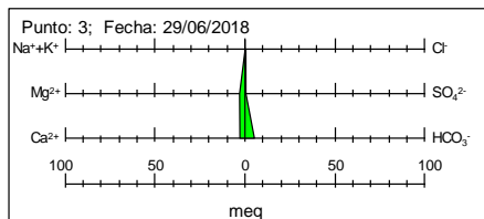
Figura 11. Diagrama del Manantial Malena del Encaño
