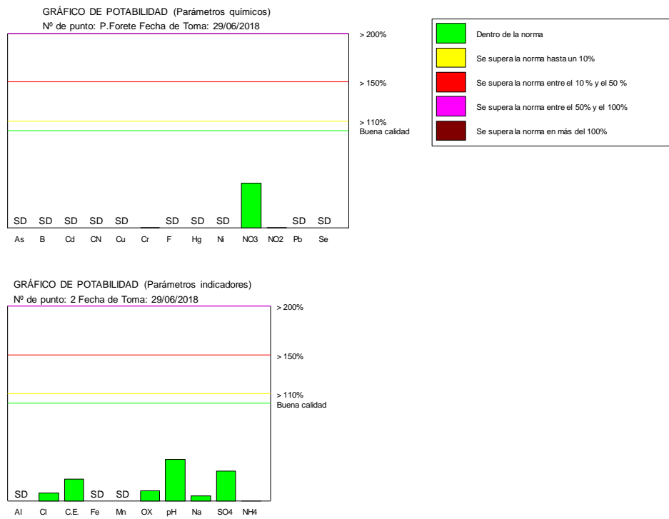
Figura 14. Gráfico de potabilidad del Pozo Forete
