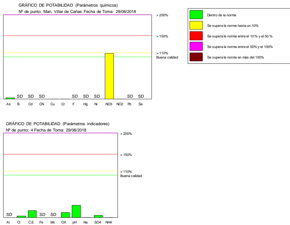
Figura 16. Gráfico de potabilidad del manantial Villar de Cañas
