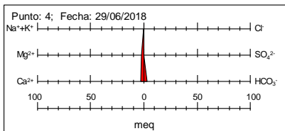
Figura 12. Diagrama de Stiff del manantial Villar de Cañas
